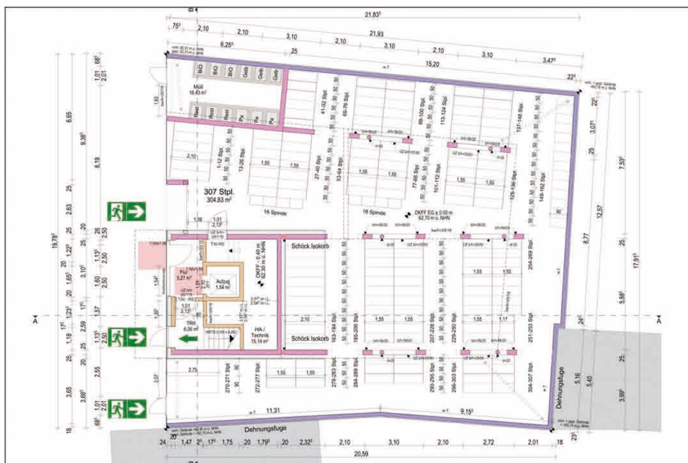
Grundriss EG
