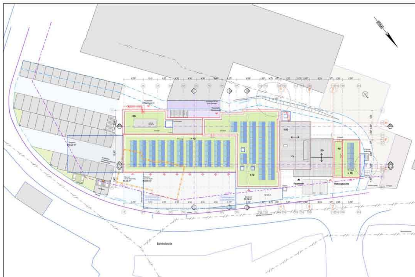
Lageplan
