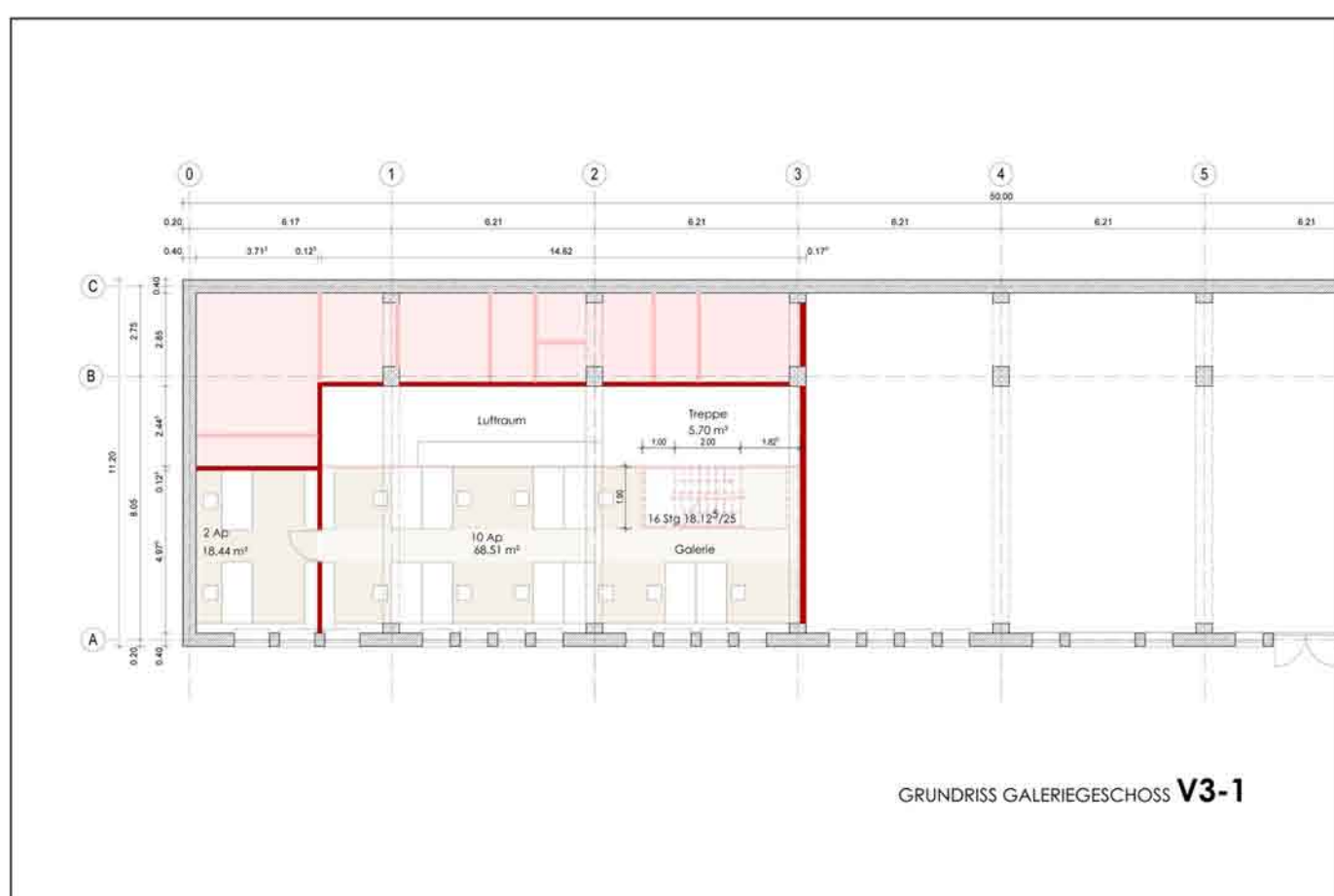
Grundriss Galeriegeschoss
