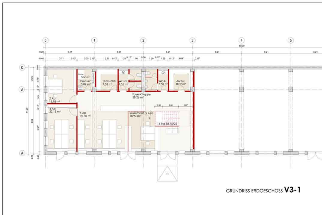
Grundriss Erdgeschoss
