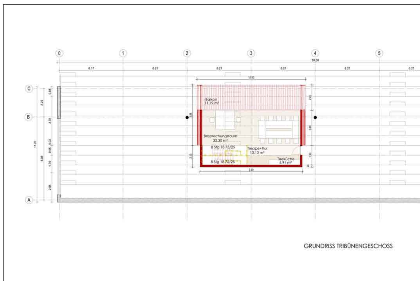
Grundriss Tribünengeschoss
