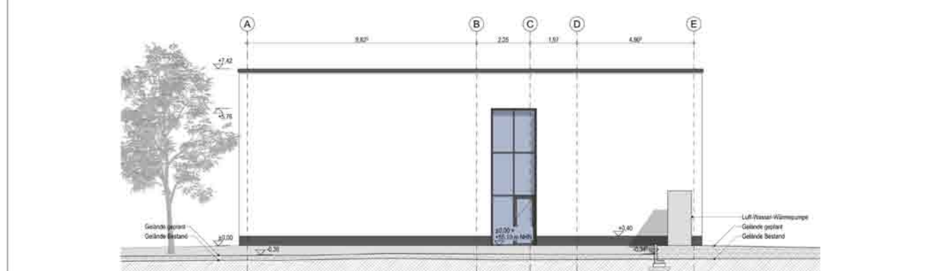
Ansicht Nord
