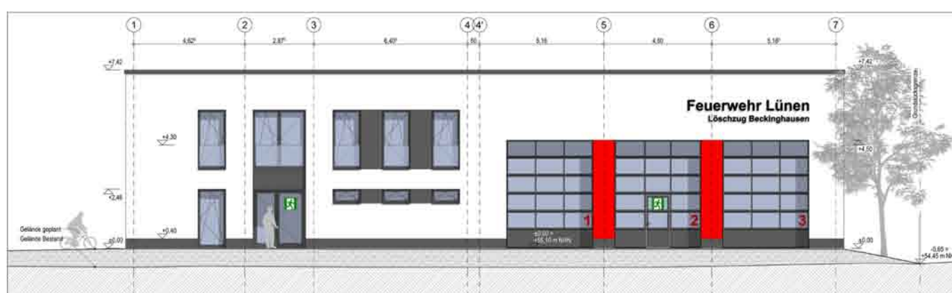
Ansicht Ost
