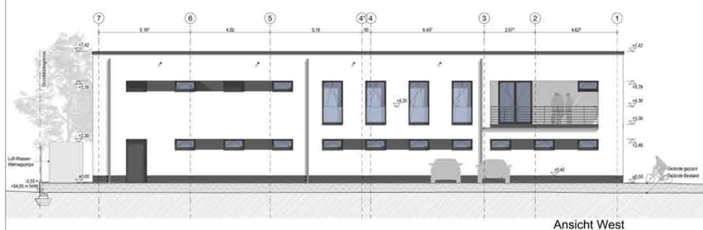
Ansicht West
