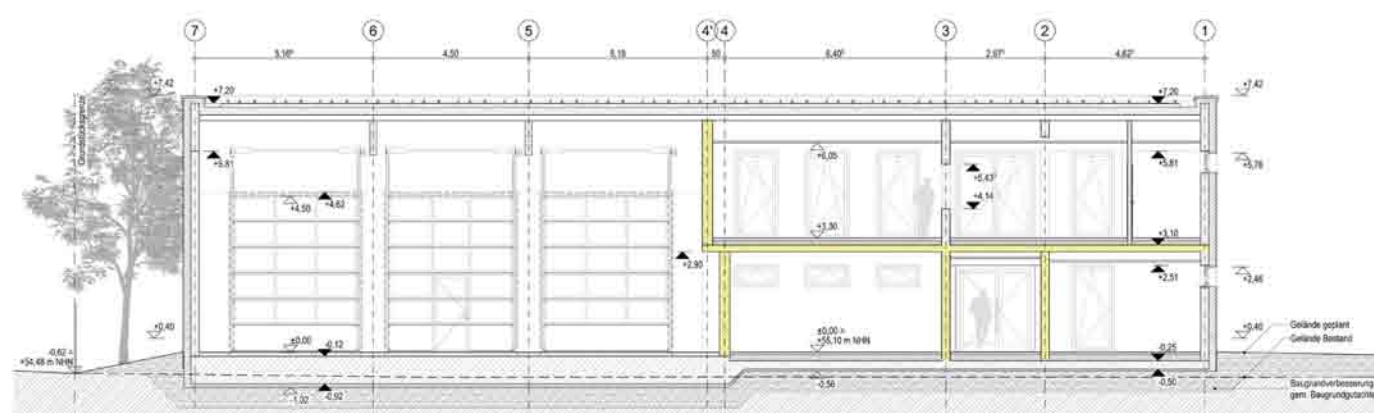
Schnitt D-D
