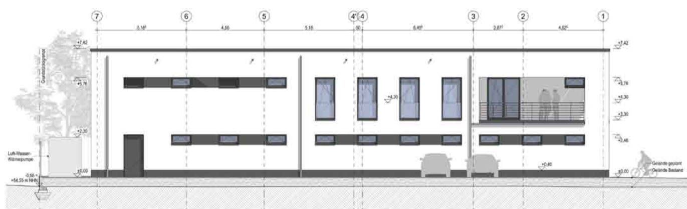
Ansicht West
