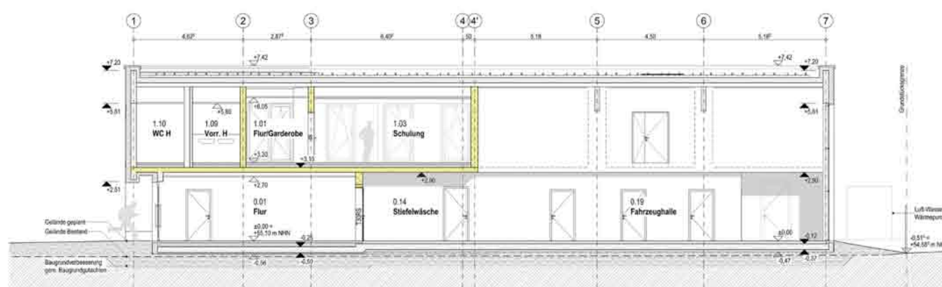
Schnitt B-B
