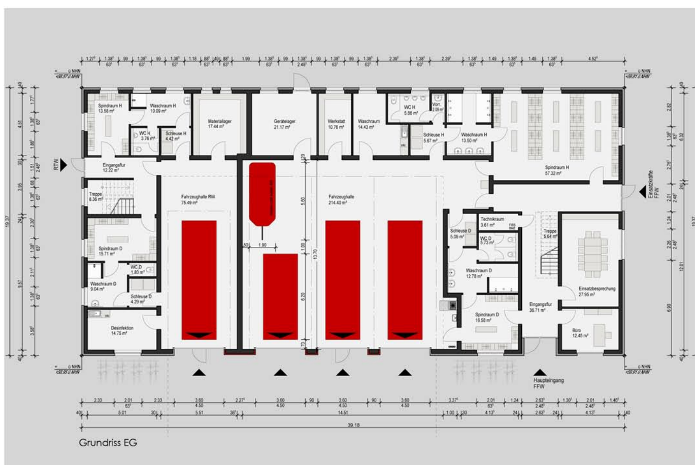
Grundriss EG
