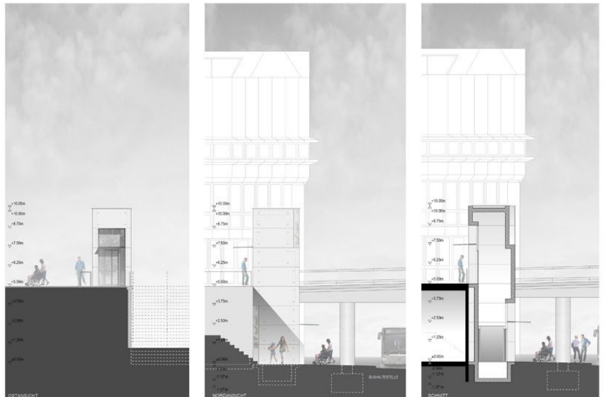
Ostansicht Nordansicht Schnitt
