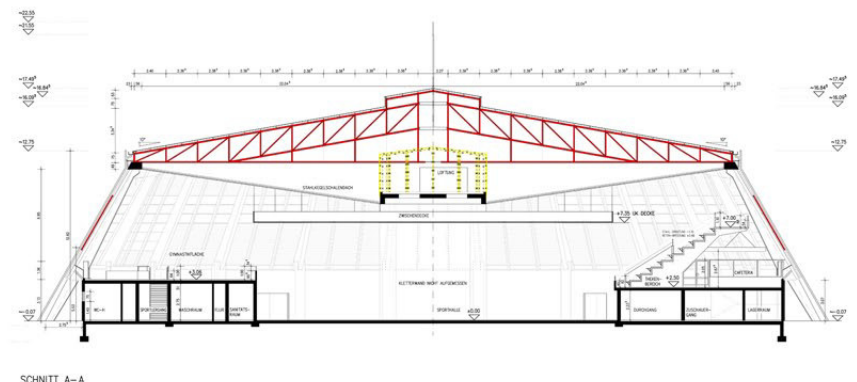
SCHNITT A-A
