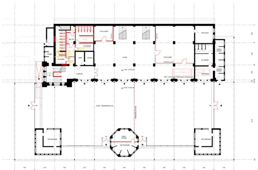
Grundriss EG
