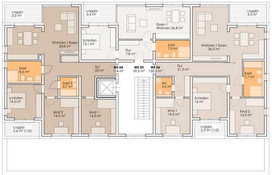
Grundriss Regelgeschoss
