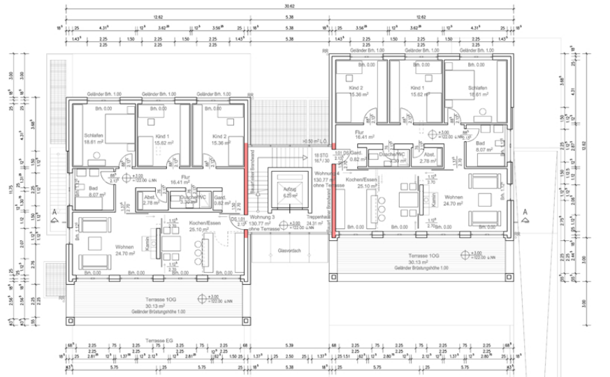
Grundriss
