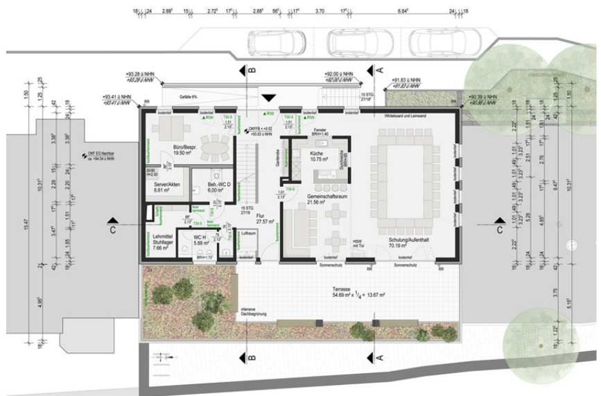
Grundriss OG
