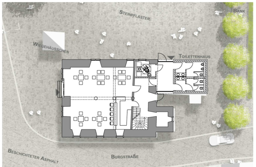
Grundriss EG
